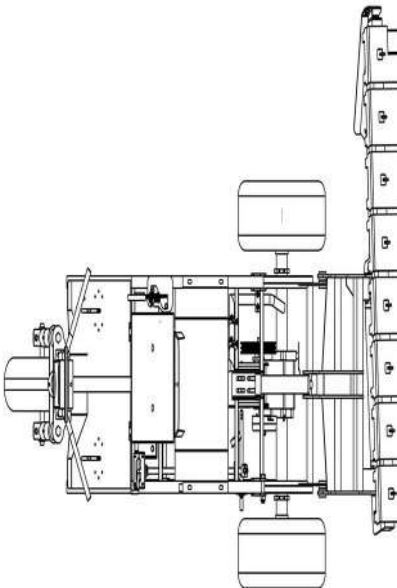
Tampak Atas
