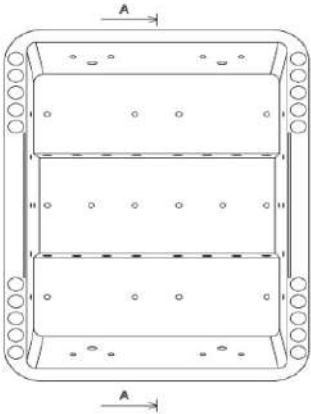
TAMPAK DATAR ATAS
