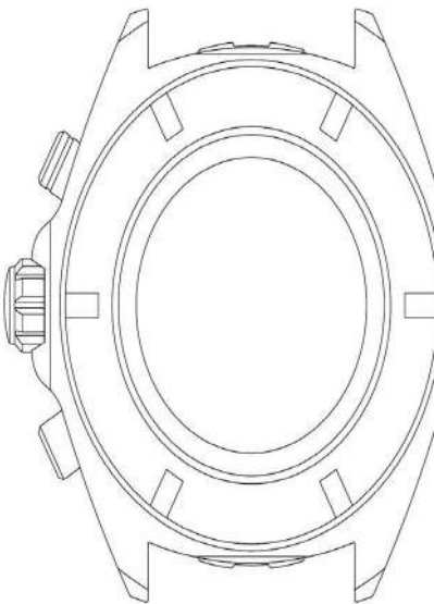
Tampak Belakang
