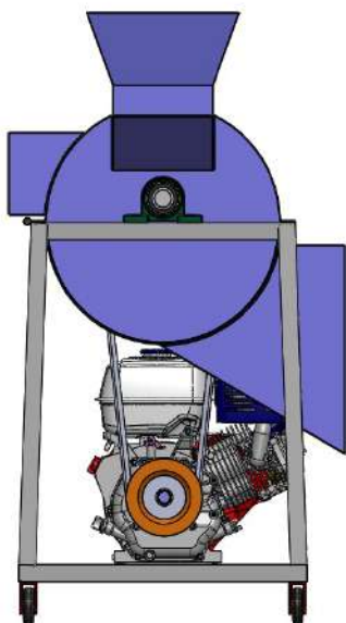
Tampak Depan
