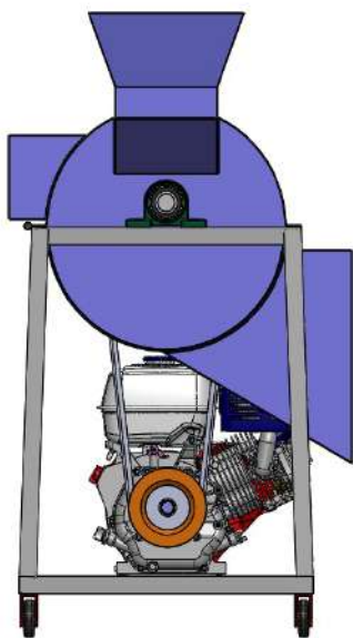
Tampak Depan
