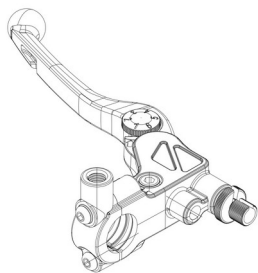
Tampak Perspektif
