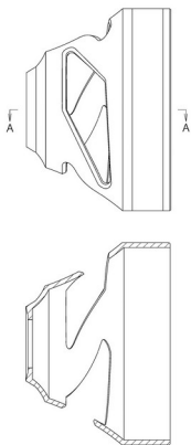
Tampak Depan
