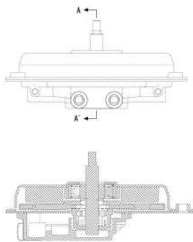
Tampak Depan
