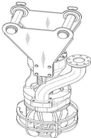
Tampak Perspektif
