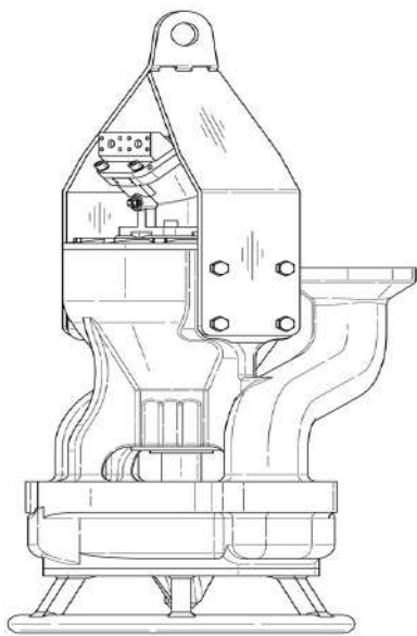
Tampak Depan
