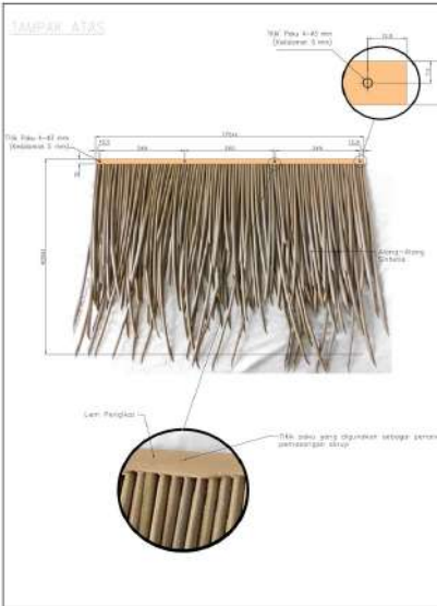
Tampak Atas
