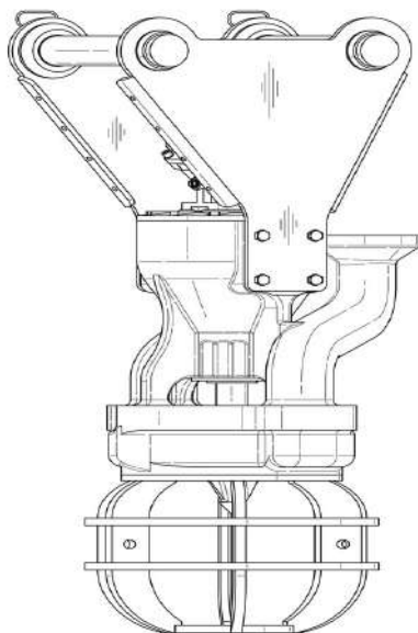
Tampak Depan
