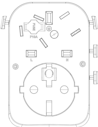
Tampak Belakang
