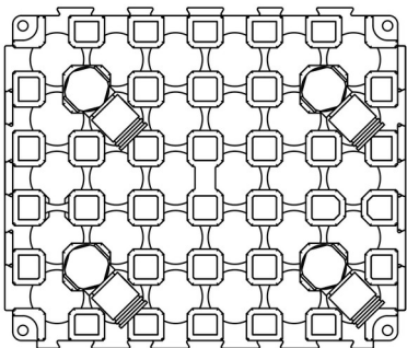
Tampak Atas
