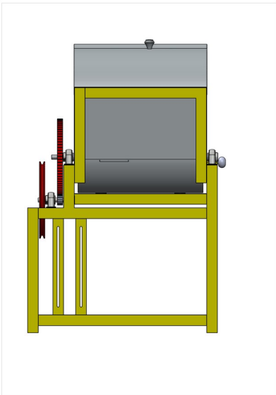
Tampak Belakang
