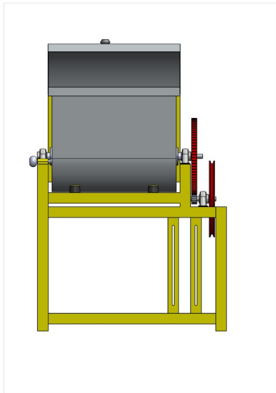
Tampak Depan
