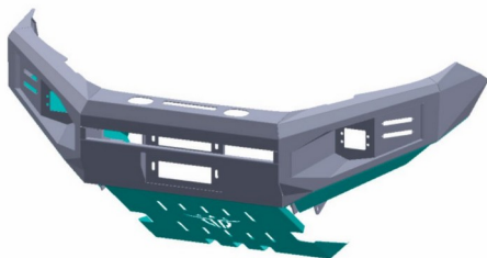
Tampak Perspektif
