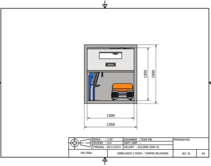
Tampak Belakang
