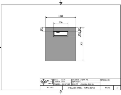
Tampak Depan
