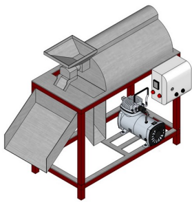
Tampak Perspektif
