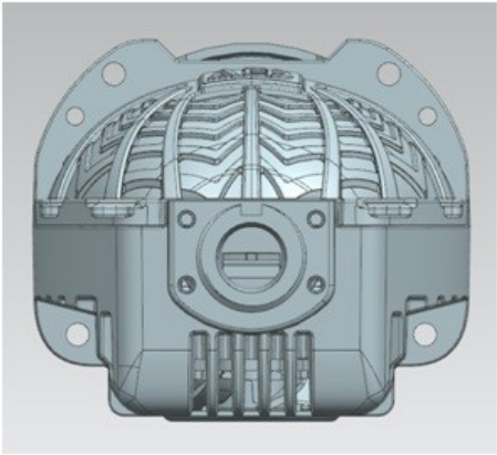
Tampak Belakang
