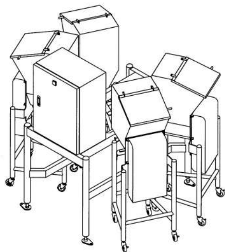
Tampak Perspektif
