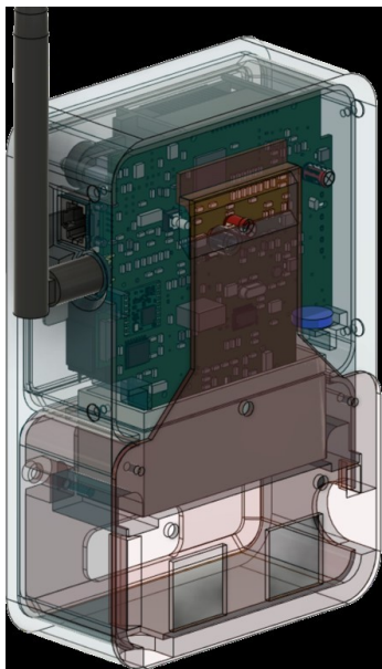
Tampak Perspektif
