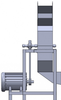
TAMPAK BELAKANG
