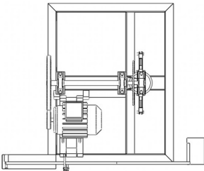
TAMPAK ATAS
