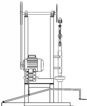
TAMPAK DEPAN
