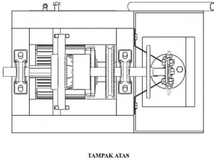
TAMPAK ATAS
