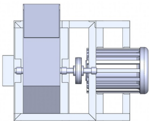
TAMPAK ATAS
