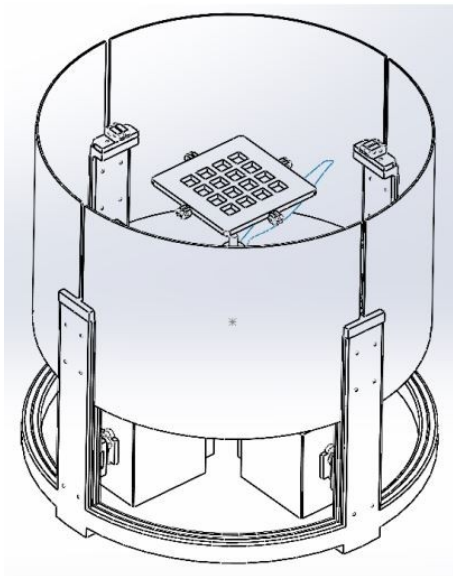
Tampak Depan
