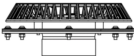
Tampak Depan
