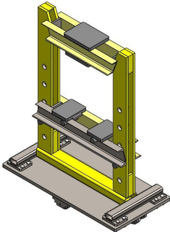
Tampak Perspektif
