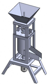
TAMPAK PERSPEKTIF
