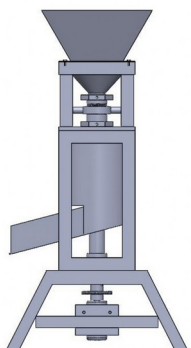
TAMPAK BELAKANG
