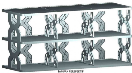
Tampak Perspektif
