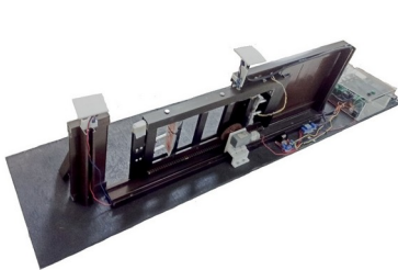
Tampak Perspektif
