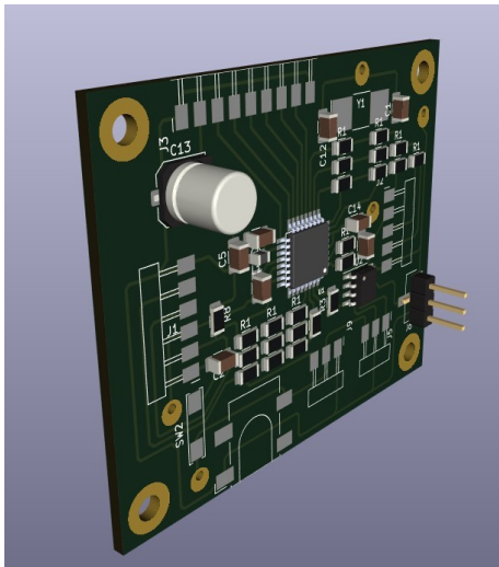
Tampak Perspektif
