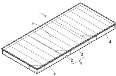
Tampak Perspektif
