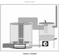
Tampak Perspektif
