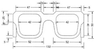
Gambar 2 : Tampak Depan
