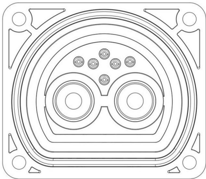
Gambar 7. TAMPAK BAWAH
