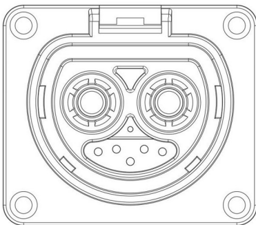
Gambar 4. TAMPAK ATAS
