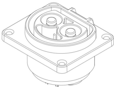
Gambar 1. TAMPAK PERSPEKTIF
