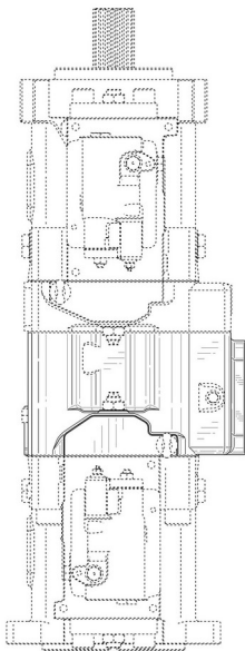
Tampak Atas
