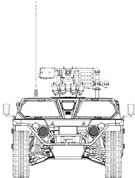
Tampak Depan
