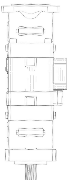
Tampak Bawah
