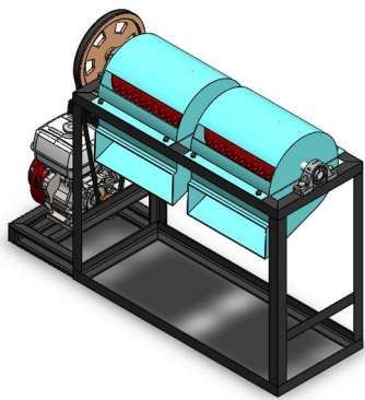
Tampak Perspektif
