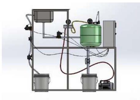
Tampak Depan
