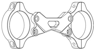
Tampak Perspektif
