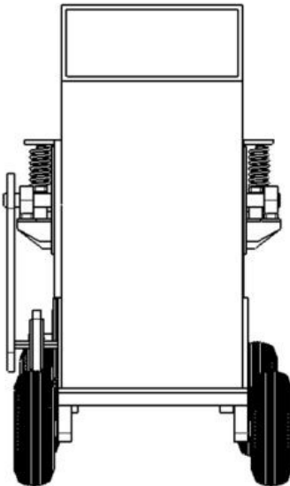
Tampak Belakang
