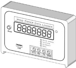
Tampak Perspektif
