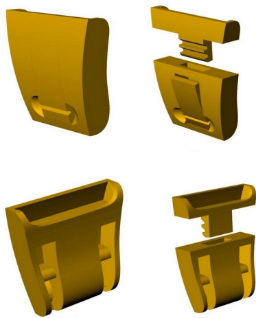
Tampak Perspektif
