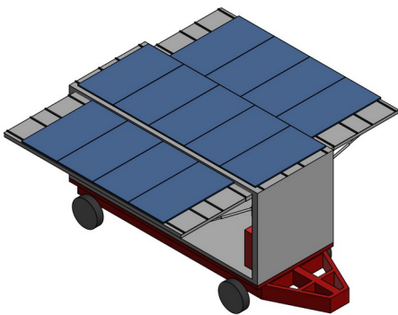
Tampak Perspektif
