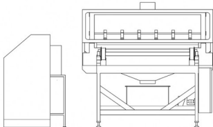
Gambar 1 – Tampak Depan
