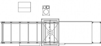
Gambar 5 – Tampak Atas
