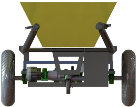
Tampak Belakang
