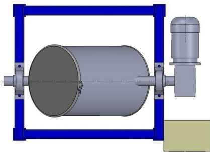
Tampak Atas
