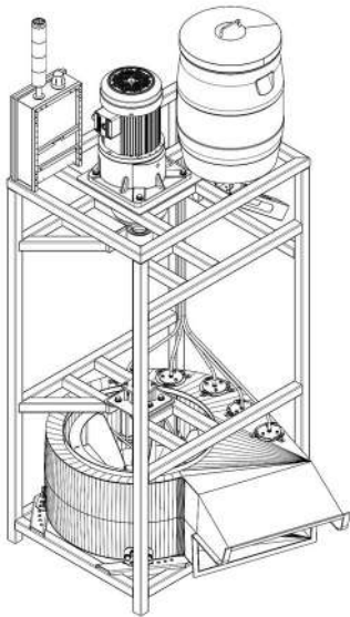
Tampak Perspektif
