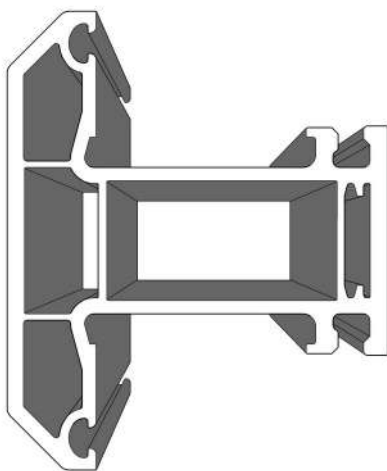
Tampak Belakang
