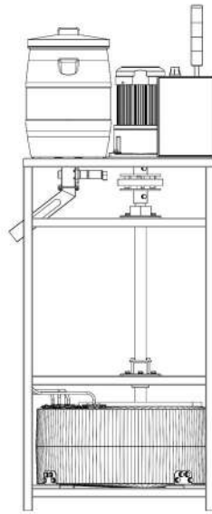
Tampak Belakang
