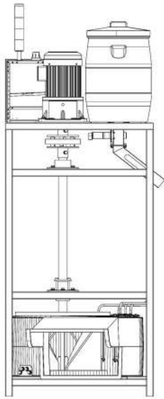
Tampak Depan
