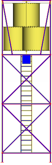
Tampak Belakang
