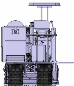
Tampak Belakang
