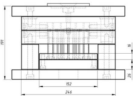
Tampak Belakang
