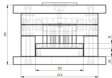
Tampak Depan
