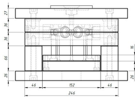
Tampak Depan
