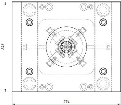
Tampak Atas
