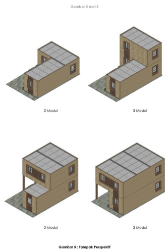
Tampak Perspektif
