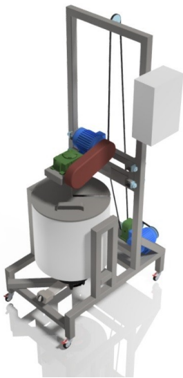
Tampak Perspektif
