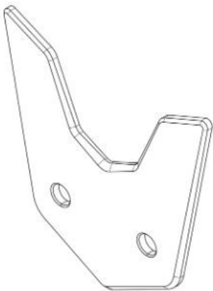
Tampak Perspektif
