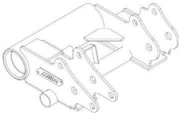
Tampak Perspektif
