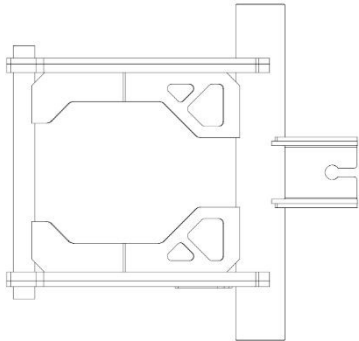
Tampak Bawah
