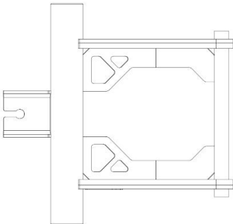
Tampak Atas
