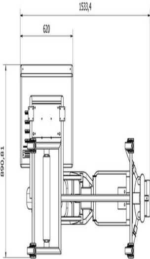
Tampak Bawah
