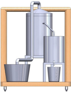
Tampak Depan
