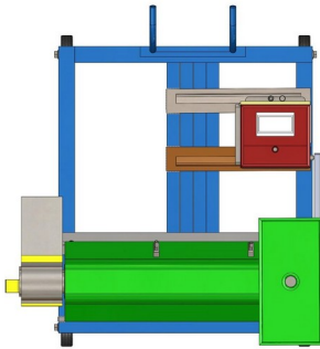
Tampak Atas
