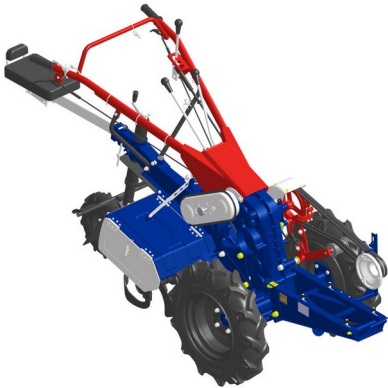
Tampak Perspektif
