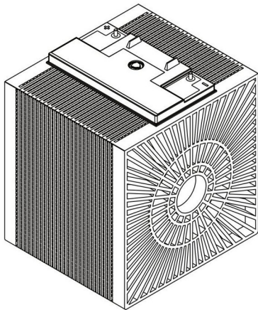
Tampak Perspektif
