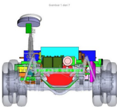
Gambar 1: Tampak Depan
