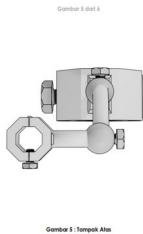
Tampak Atas
