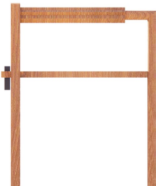
Gambar 2: Tampak Belakang
