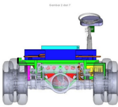
Gambar 2: Tampak Belakang
