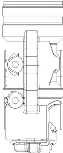
Tampak Belakang
