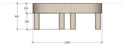
Tampak Belakang
