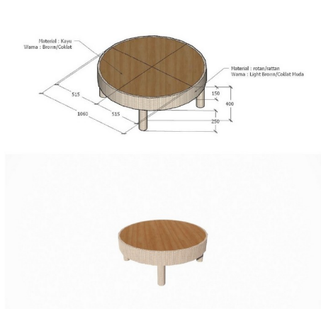
Tampak Perspektif
