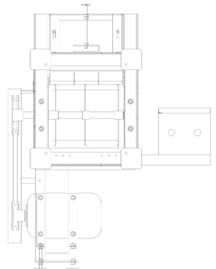
Tampak Bawah
