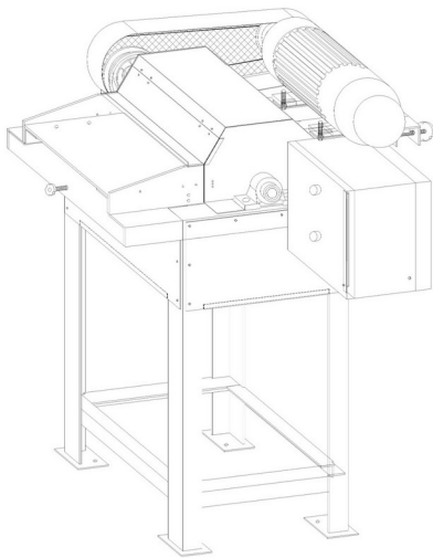
Tampak Perspektif
