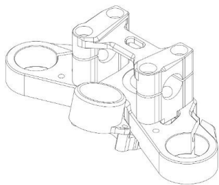
Tampak Perspektif
