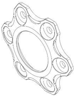
Tampak Perspektif
