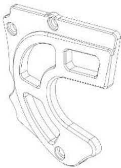
Tampak Perspektif
