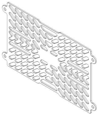
Tampak Perspektif
