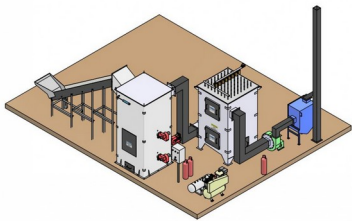
GAMBAR PERSPEKTIF
