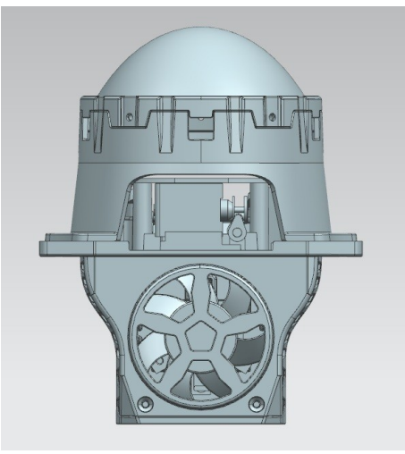
Tampak Bawah
