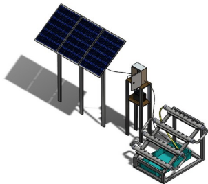
Tampak Perspektif
