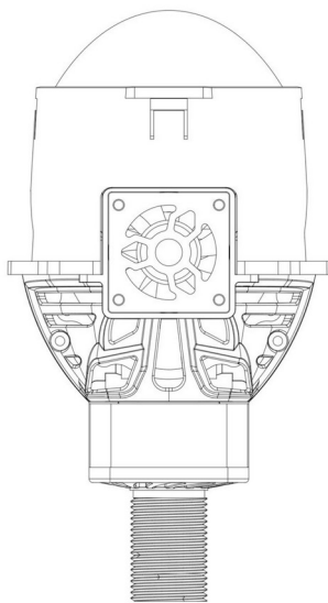
Tampak Atas
