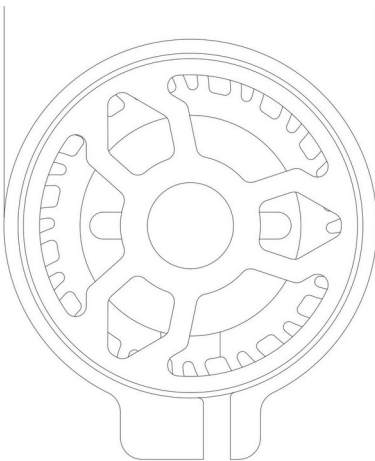
Tampak Atas
