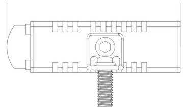
Tampak Bawah
