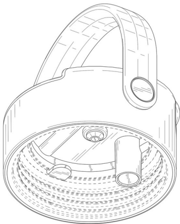
Tampak Perspektif
