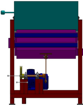
Tampak Belakang
