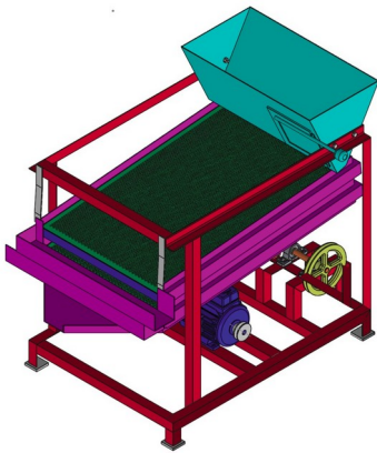
Tampak Perspektif
