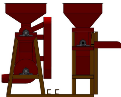
Tampak Belakang
