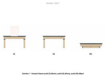
Tampak Depan
