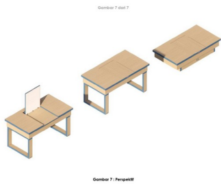
Tampak Perspektif
