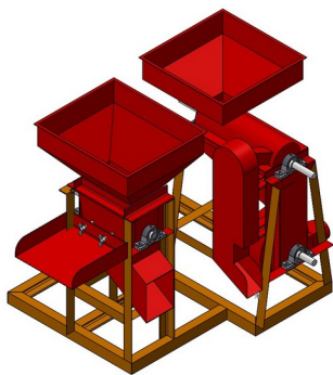
Tampak Perspektif
