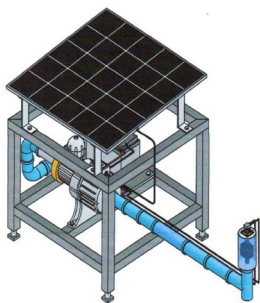
Tampak Perspektif
