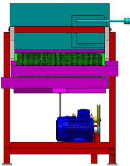
Tampak Depan
