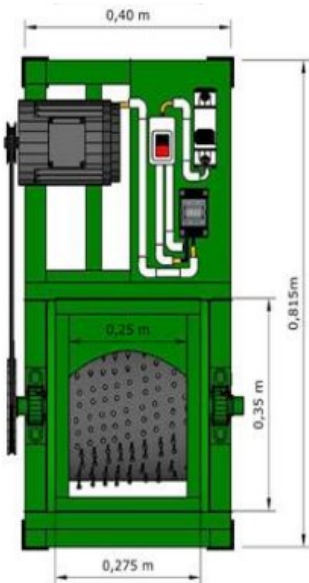
Tampak Atas
