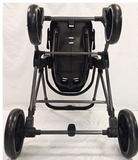
Tampak Bawah
