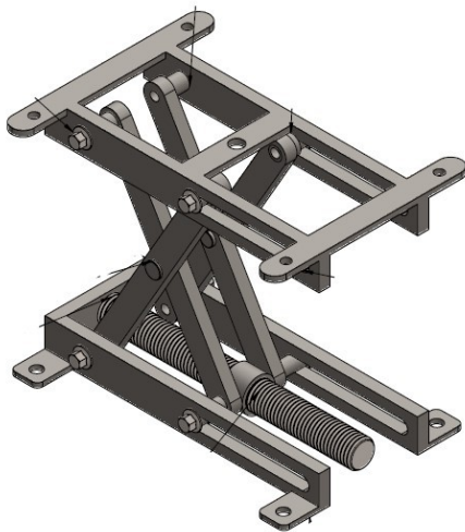
Tampak Perspektif
